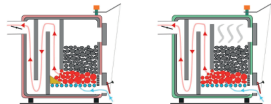
Kocioł dolnego spalania
