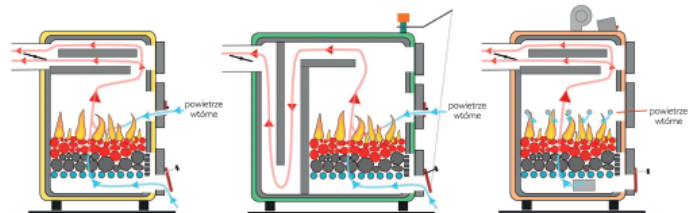
Kocioł z poziomym wymiennikiem
