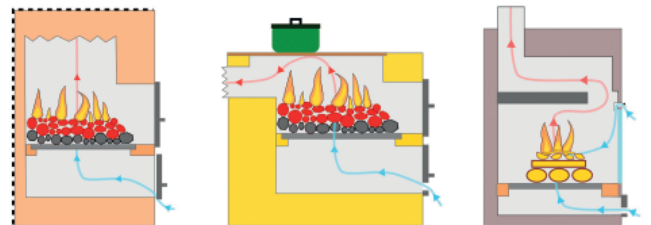
Piec kaflowy
