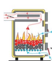
Kocioł z poziomym wymiennikiem
