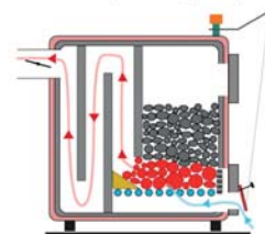
Kocioł dolnego spalania
